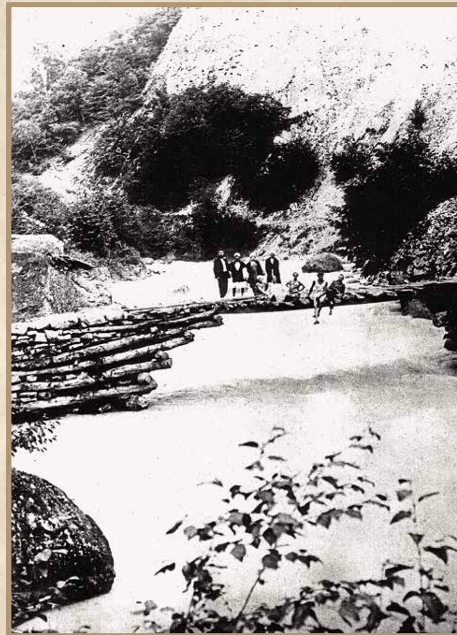
♣ Мост горской системы на бревенчатых опорах через Черек Балкарский
